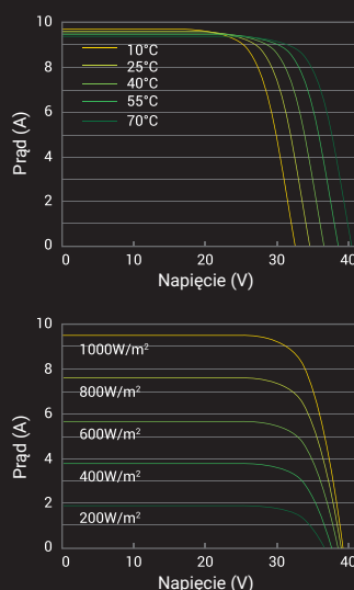
Krzywa prądowo-napięciowa: (A-HCM340)
